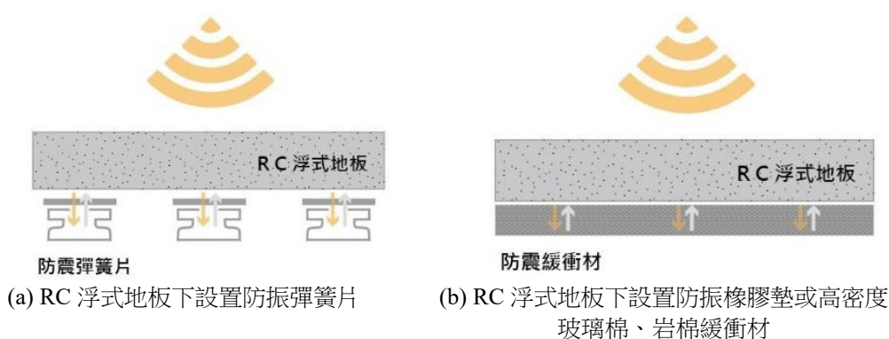
圖 7-18 樓板表面材(含緩衝材)應用例
